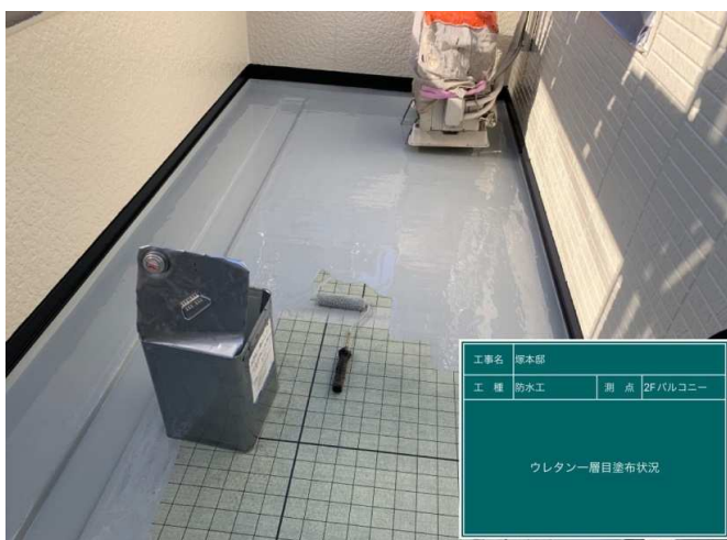
47 ベランダ ウレタン1層目 施工中
