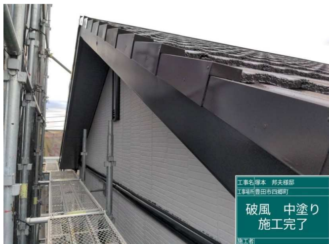
20 破風板 中塗り 施工完了
