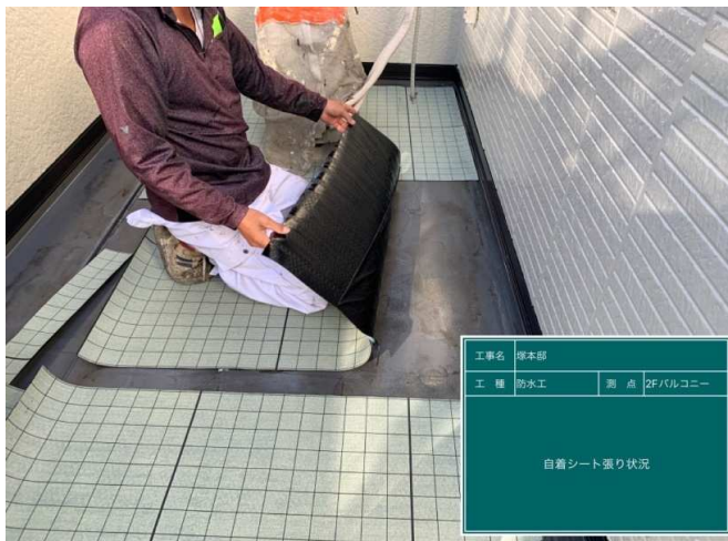
45 ベランダ 自着シート貼り 施工中
