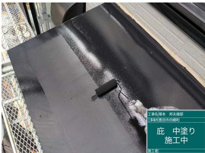
29 庇 中塗り 施工中
