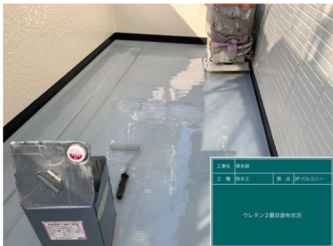
49 ベランダ ウレタン2増目 施工中
